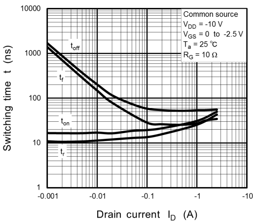
Fig. 7.11 t - I_D
