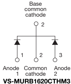
TO-263AB (D 2 PAK)
