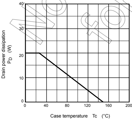
P_D - T_c
