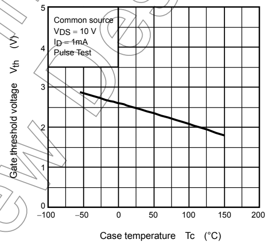
V_{th} - T_c
